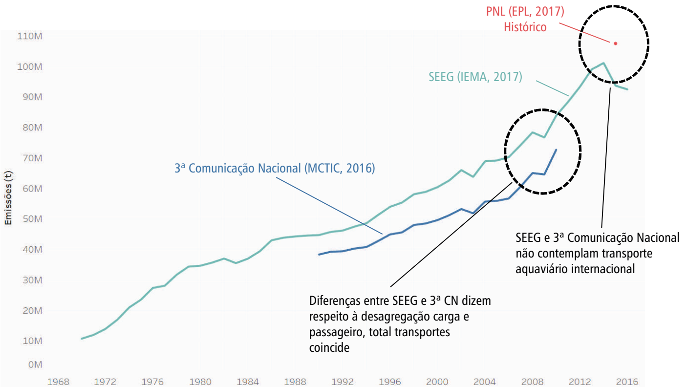
Histórico de emissões de GEE no transporte de cargas (tCO 2 e ou tCO 2 )
