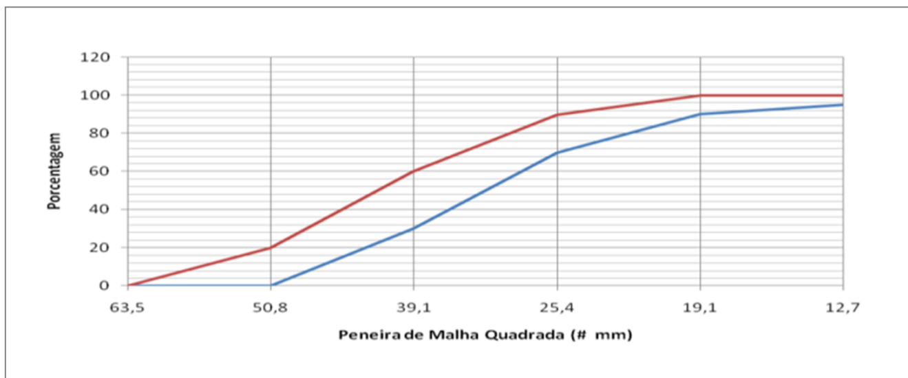
Figura 1 - Granulometria de Pedra Britada para Lastro – Percentual Retido
